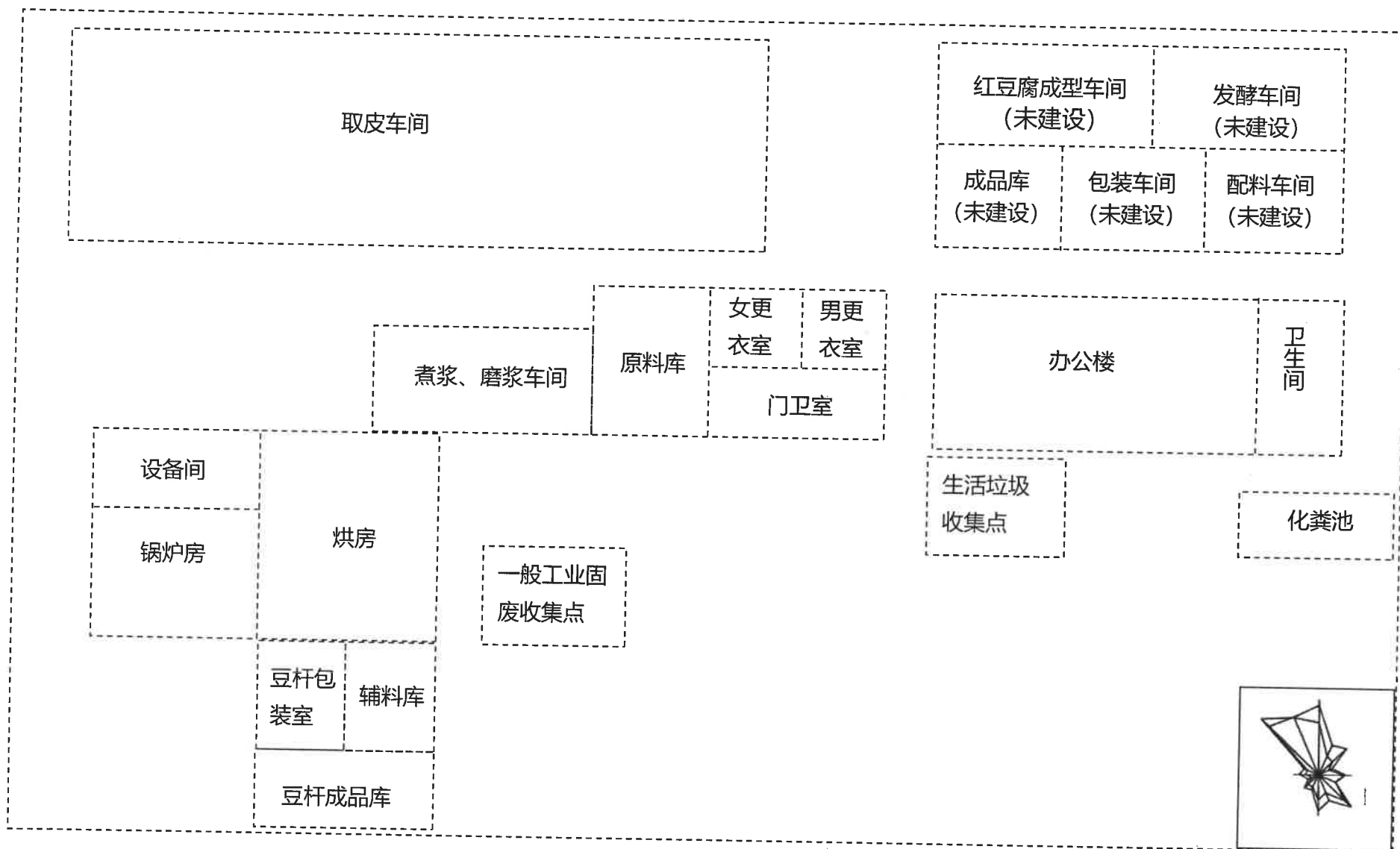
附图3 项目总平面布置及环保设施分布图
